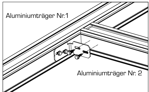
Verbindung mit waagrechttem Winkel
