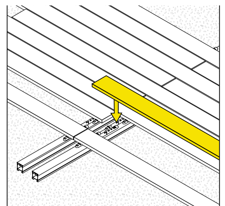
Doppelte Unterkonstruktion
