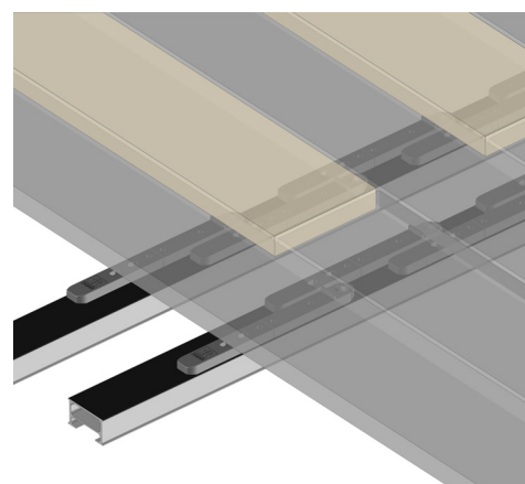
Doppelte Unterkonstruktion
