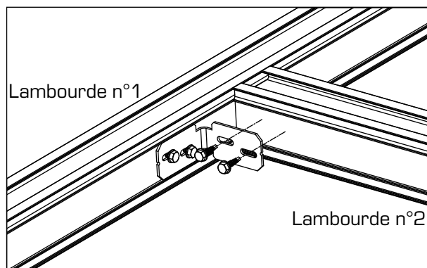
Assemblage avec équerrre horizontale
