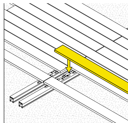
Double lambourdage
