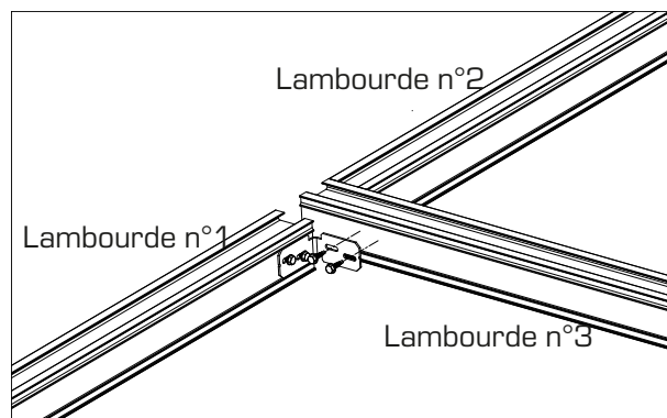
Cas particulier : aboutage avec équerrre horizontale
