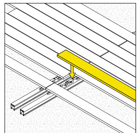
Doppelte Unterkonstruktion
