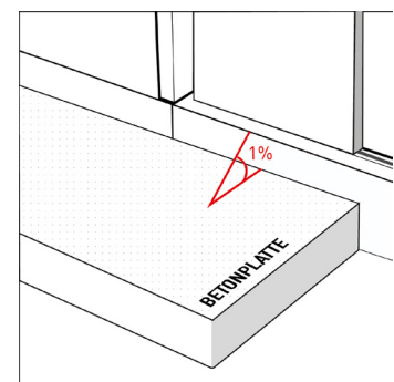
Mindestens 1% Gefälle
