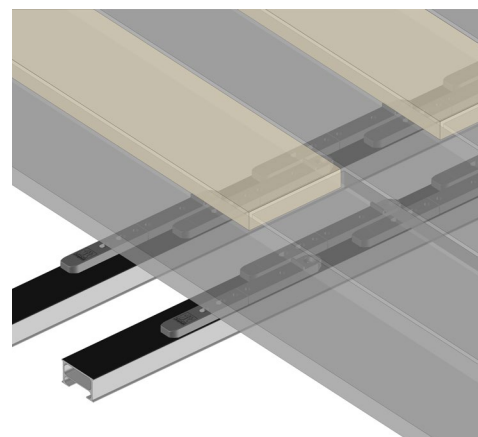
Doppelte Unterkonstruktion
